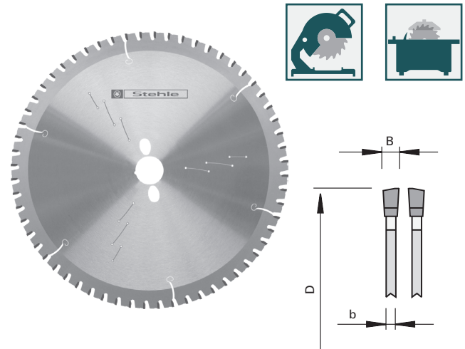
Unisteel Metall-Kapp-Kreissägeblätter HW, „F-WFA“
