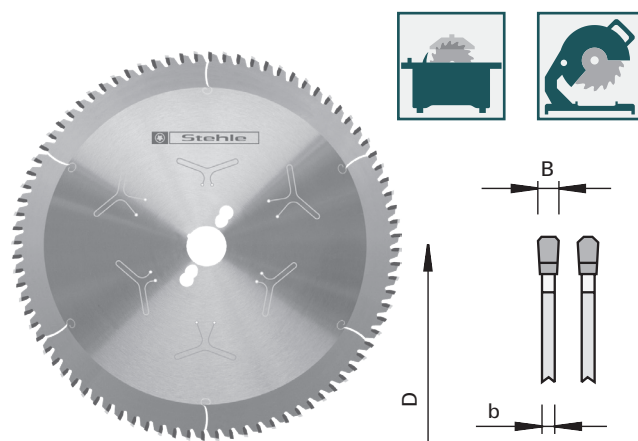
KKS - plástico duro positivo & *negativo Discos de sierra HW para perfiles de plástico extremadamente duros, „TR-F-FA“
