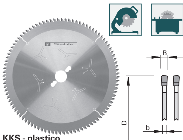
KKS - plástico Discos de sierra HW para perfiles de plástico, „WS-FA“
